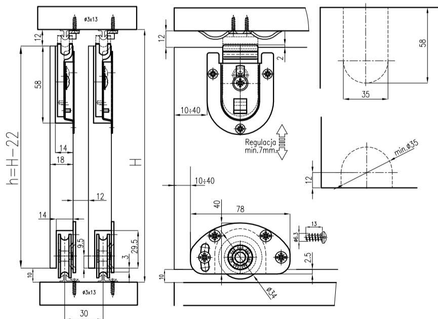
montaż okuc wewnątrz płyty
