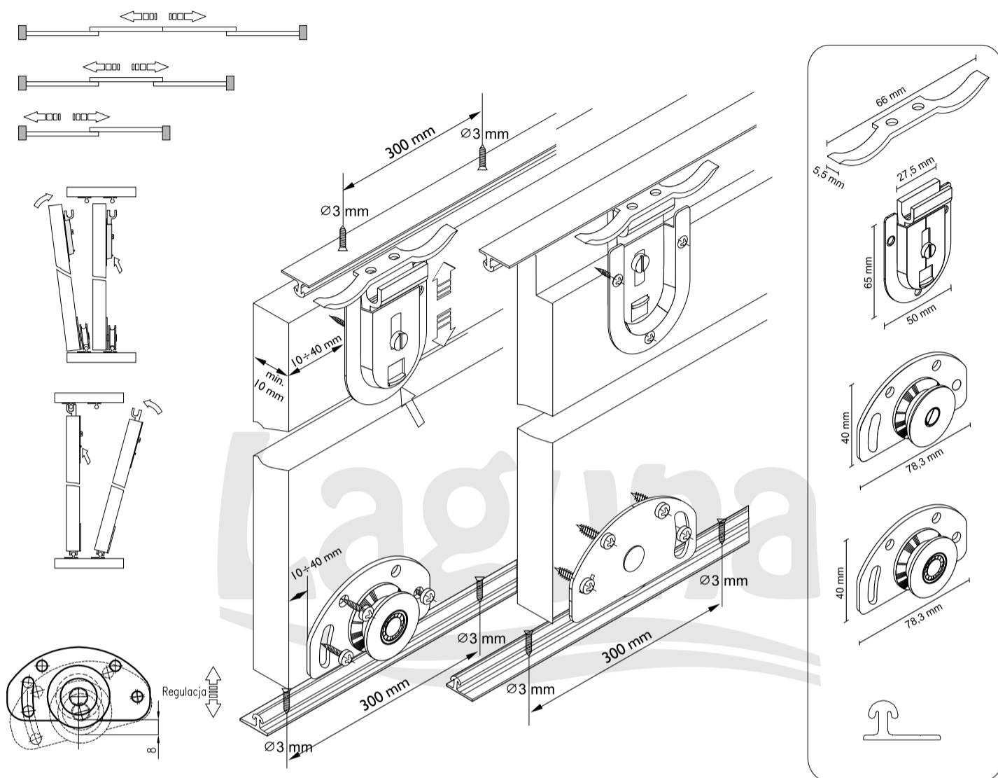
montaż okuc wewnątrz płyty
